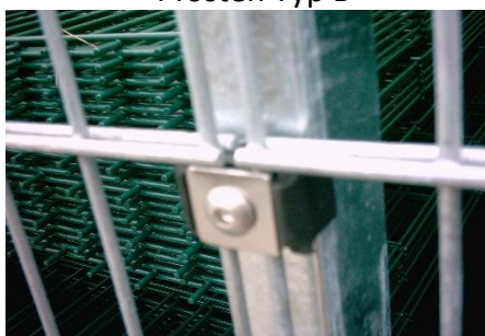
Eckverbinder
